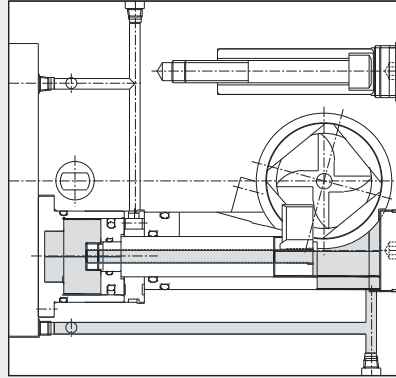
45° INDEX
