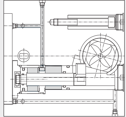
90° INDEX
